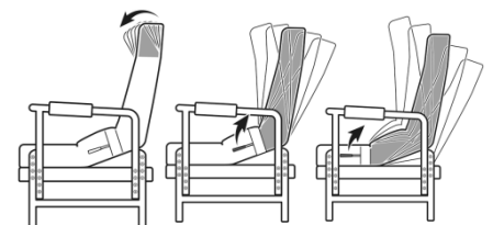
ヘッドレスト・背もたれ・座面(後部)の角度調整
